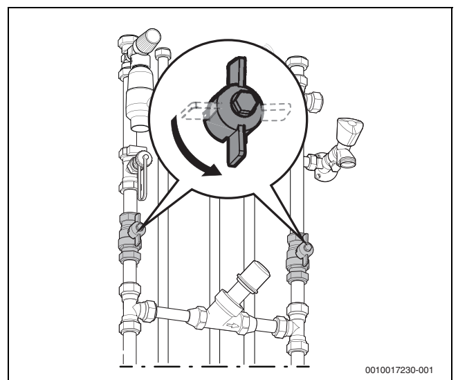
Afb. 4 Serviceafsluiters
