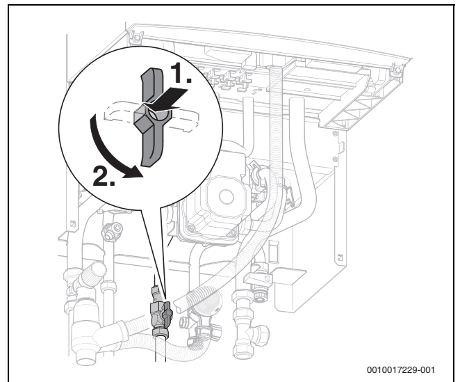
Afb. 3 Gaskraan
