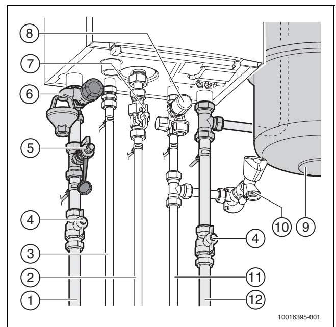
Afb. 2 Overzicht aansluitingen
