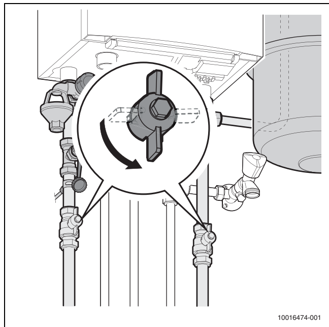
Afb. 4 Serviceafsluiters
