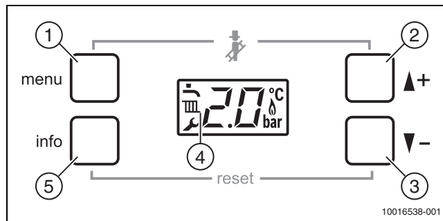
Afb. 6 Bedieningspaneel
