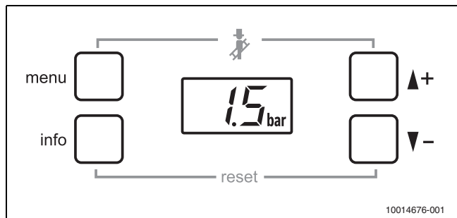
Afb. 5 Aflazen cv-waterdruk
