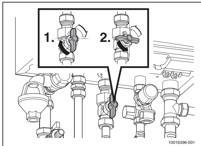
Afb. 3 Gaskraan
