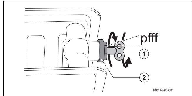
Afb. 8 Ontluchten radiator
